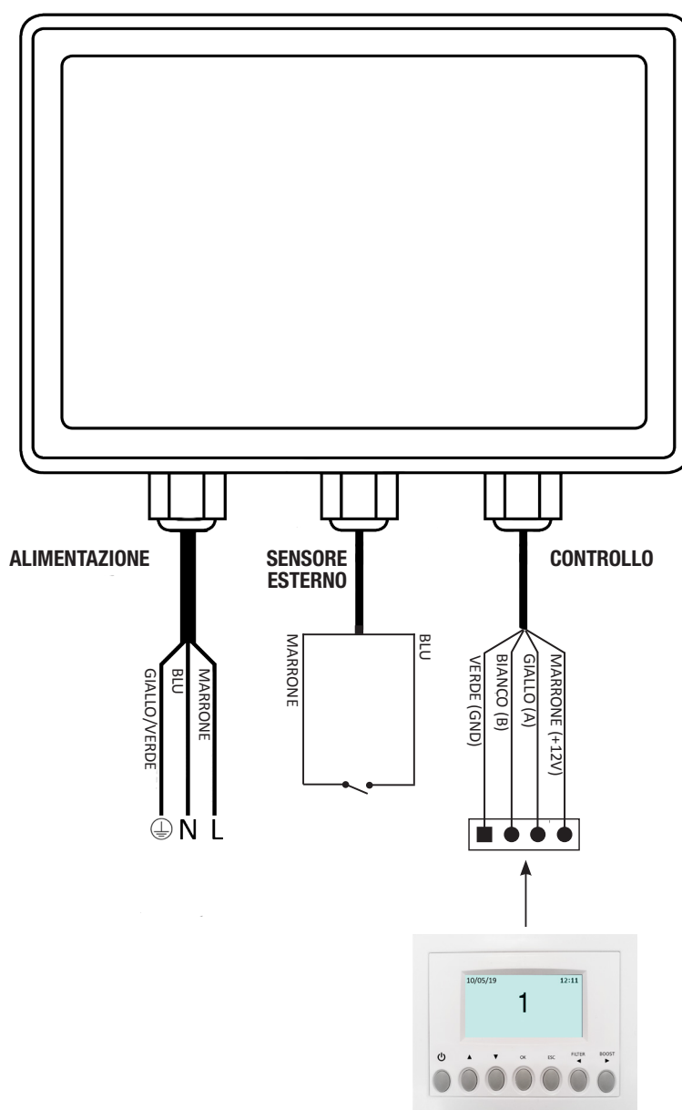
Fig. 5.g Collegamento cavi
