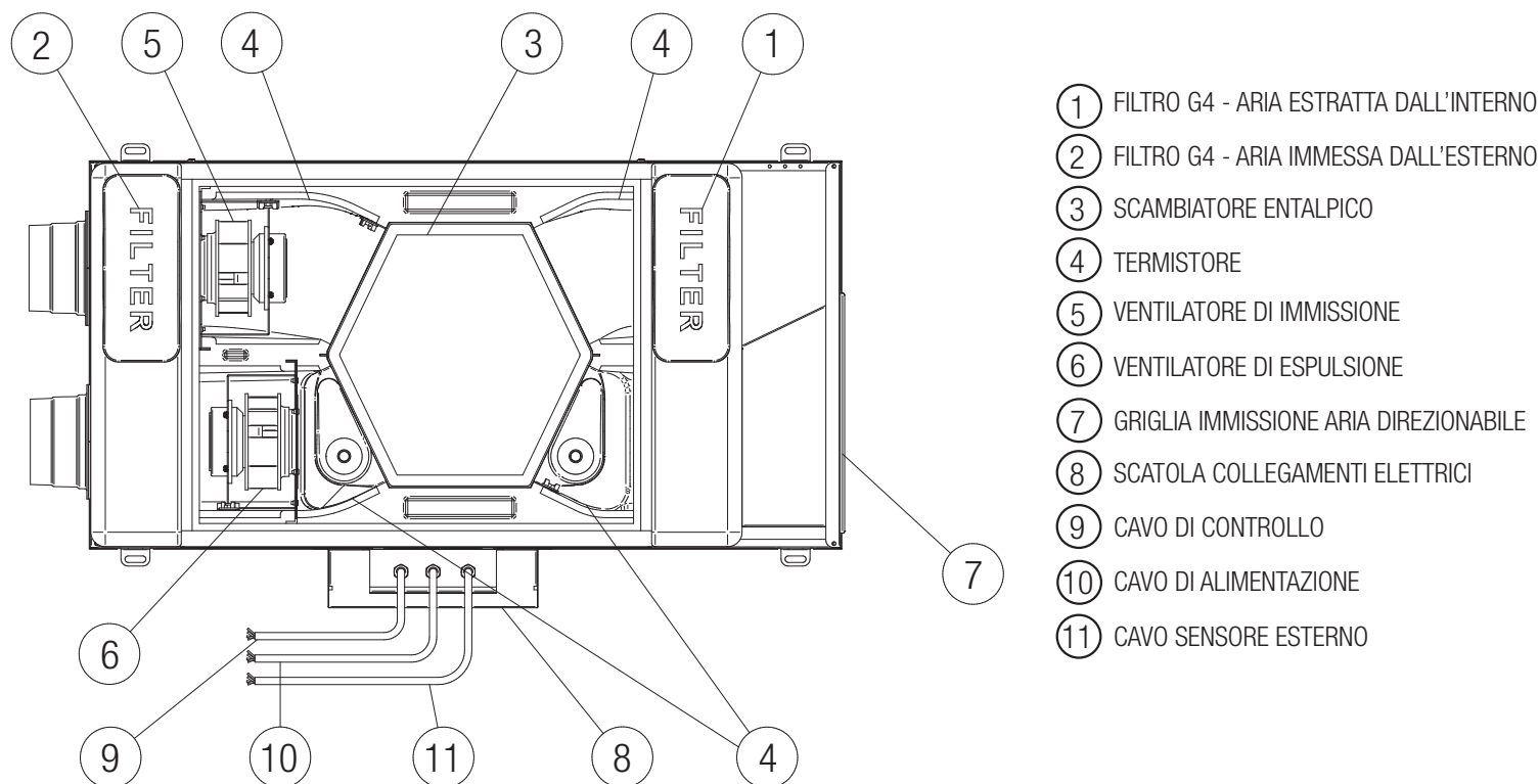
Fig. 8.a Componenti interni
