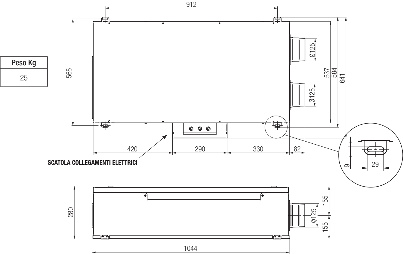
Fig.3.a Dimensioni in mm.
