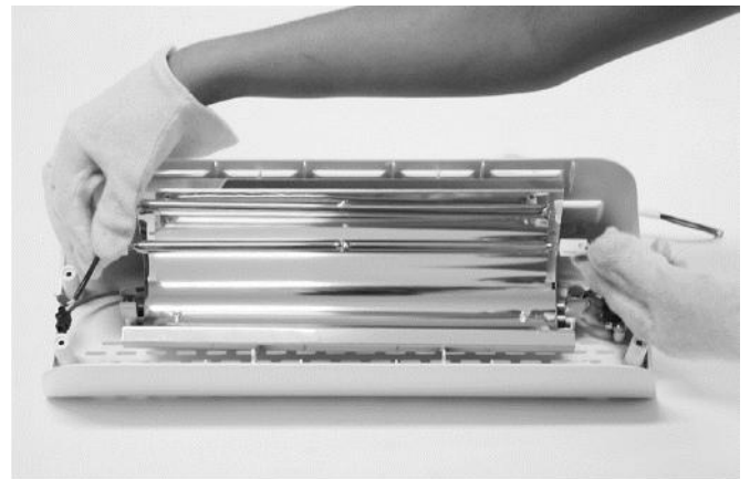
4. EXTRAER LA BOMBILLA DE LOS DOS RESORTES
