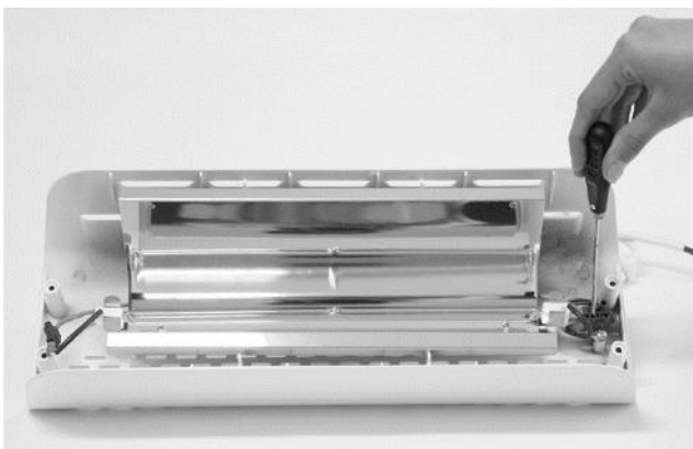
3. QUITAR LAS DOS CUBIERTAS LATERALES Y LOS DOS CABEZALES DE LA PARÁBOLA. DESATORNILLAR (EN LOS BORNES ALOJADOS EN LAS CUBIERTAS LATERALES) LOS TORNILLOS QUE SOSTIENEN LOS DOS CABLES DE LA BOMBILLA
