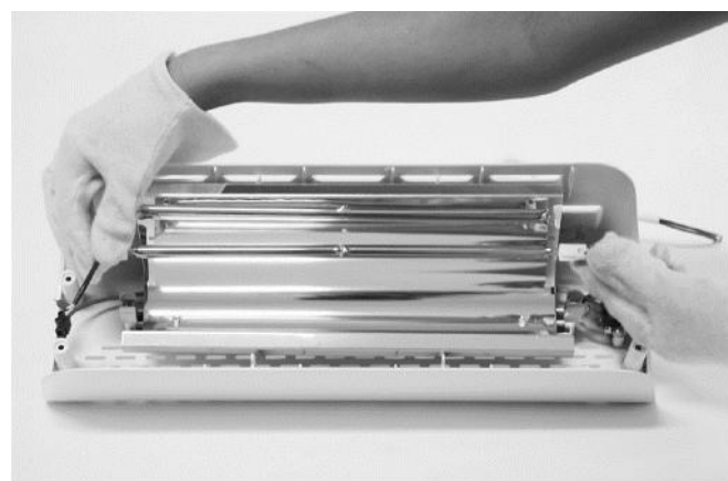
4. TOGLIERE IL BULBO DALLE MOLLETTE
