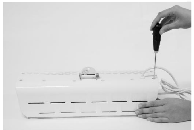
2. DESATORNILLAR LOS 4 TORNILLOS DE LA PARTE POSTERIOR
