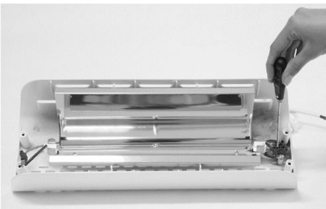
3. RETIRER LA PARTIE ANTÉRIEURE DE L'APPAREIL. DÉVISSER LES VIS DES BORNES AUXQUELLES SONT RELIÉS LES FILS D'ALIMENTATION DE L'AMPOULE.
