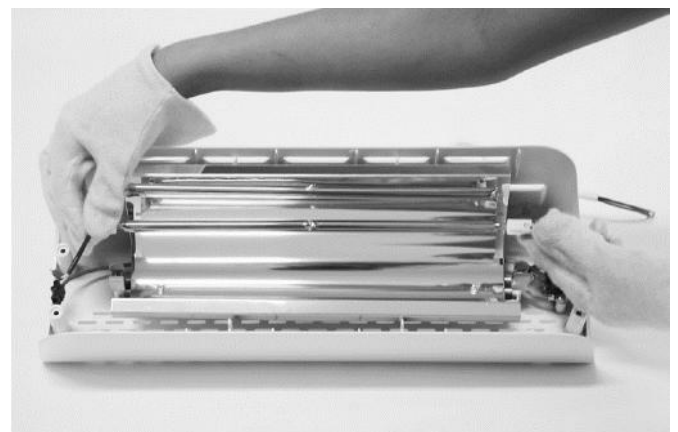
4. EXTRAIRE L'AMPOULE DES CLIPS.
