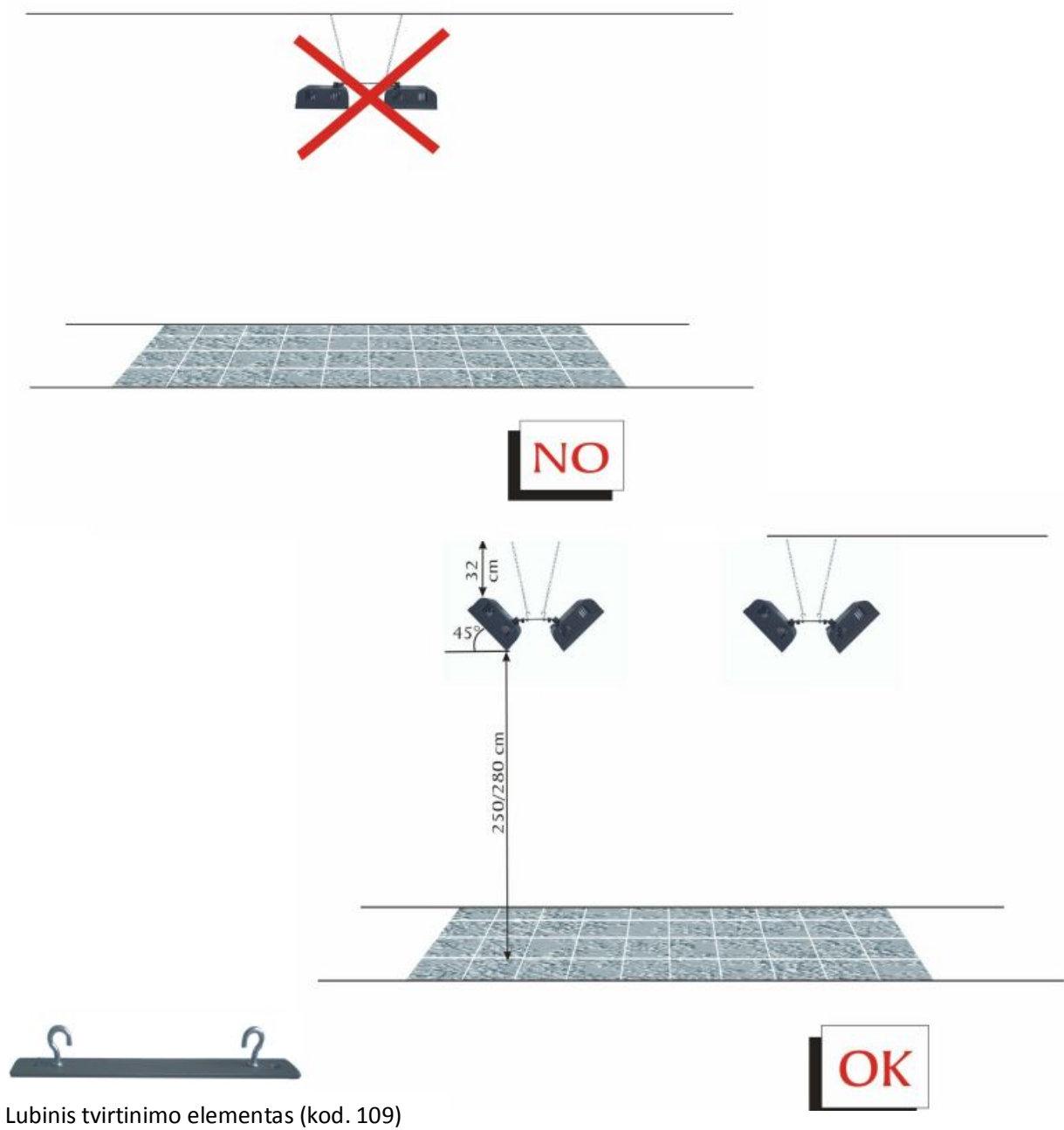
2 pav. Montavimas prie lubu - minimalūs atstumai
