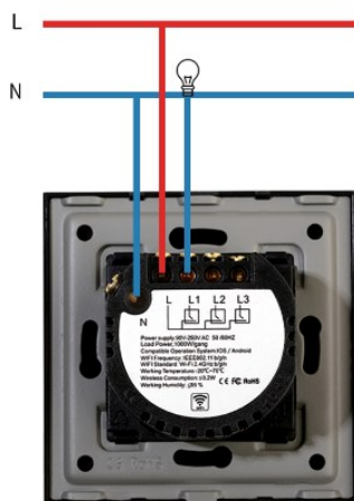
1 pav. Pagrindinio jungiklio prijungimo schema
